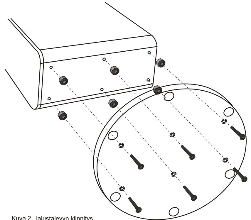
Kuva 2. jalustalevyn kiinnitys
